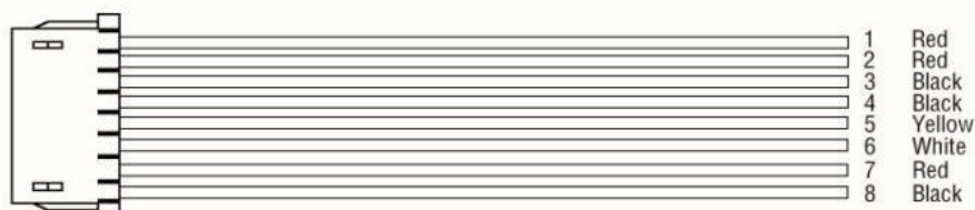
Wiring Table:
